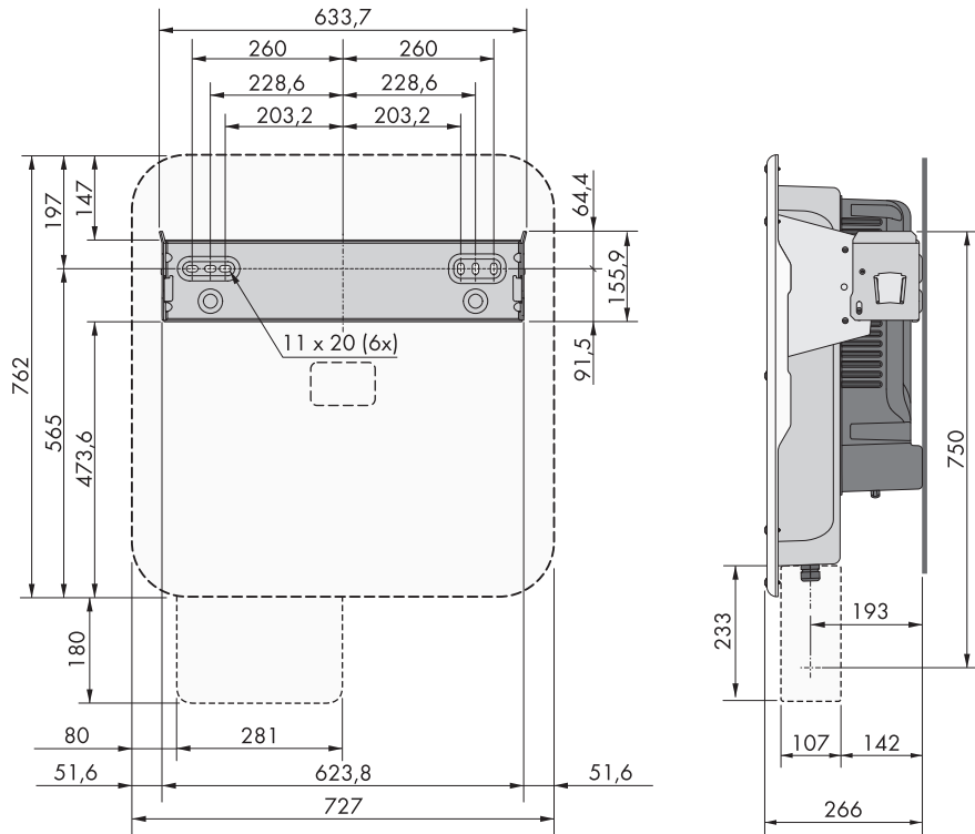
Abbeelding 6: Positie van de bevestigingspunten (afmetingen in mm)
