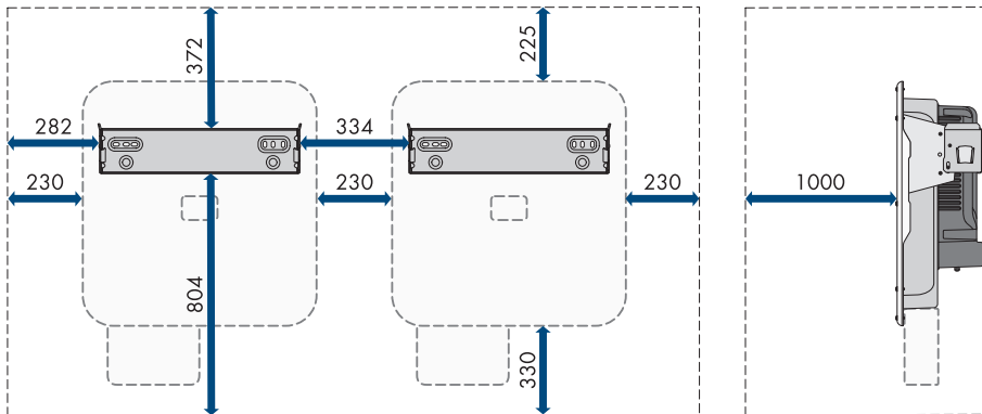
Afbeelding 7: Aanbevolen afstanden (afmetingen in mm)
