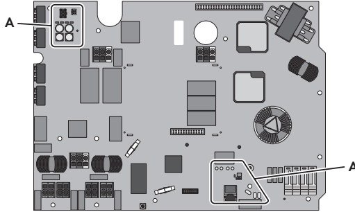
Şekil 2 : SELV devrelerinin pozisyonu
