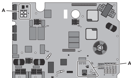
Figura 2 : Posizione dei circuiti SELV
