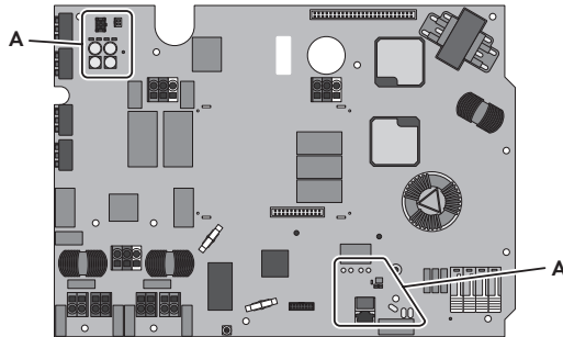
Εικόνα 2 : Θέση των κυκλωμάτων SELV
