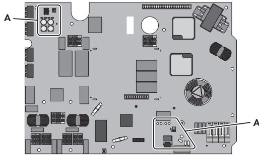
Imagen 2 : Posición del circuito SELV
