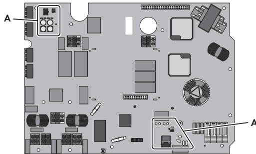
Afbeelding 2 : Positie van de SELV-circuits
