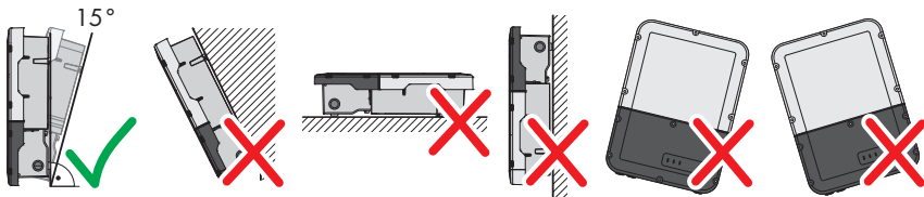
Figure 3 : Positions de montage autorisées et non autorisées
