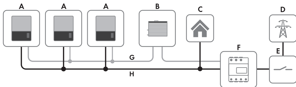
図 25 合計出力一定制限下での売電運転 / ピークカット
