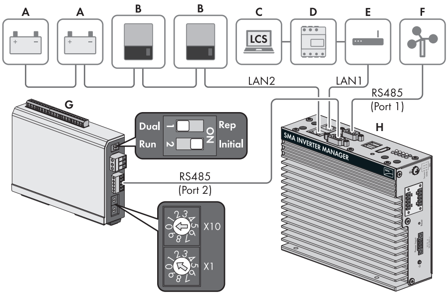
Imagen 3: Esquema de interconexión Sunny Tripower Storage 60
