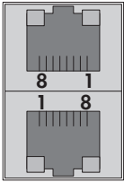
Abbildung 4: Pin-Belegung der Netzwerkbusen
