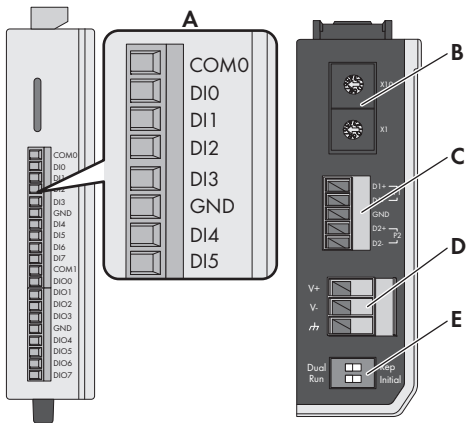
Abbildung 9: Übersicht Anschluss I/O Box
