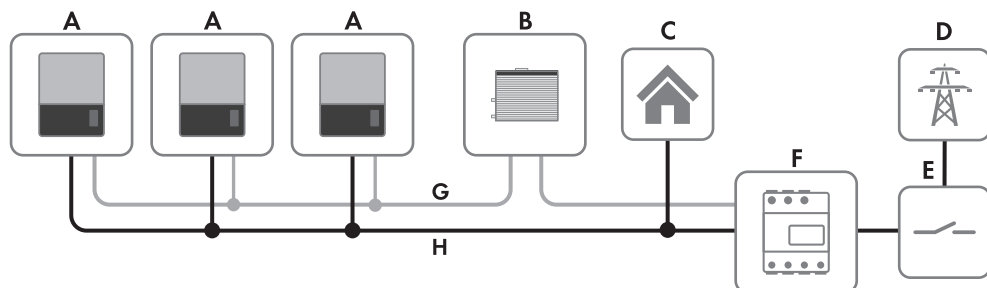
Imagen 25: Funcionamiento de inyección con Limited Export/Peak Load Shaving
