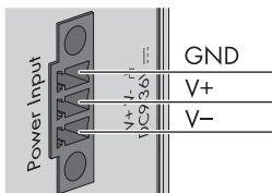
Figure 7: Affectation des broches de l'embase « Power Input » SMA recommande d'utiliser le bloc d'alimentation pour rail DIN disponible en accessoire (numéro de commande : CLCON-PWRSUPPLY)*.
