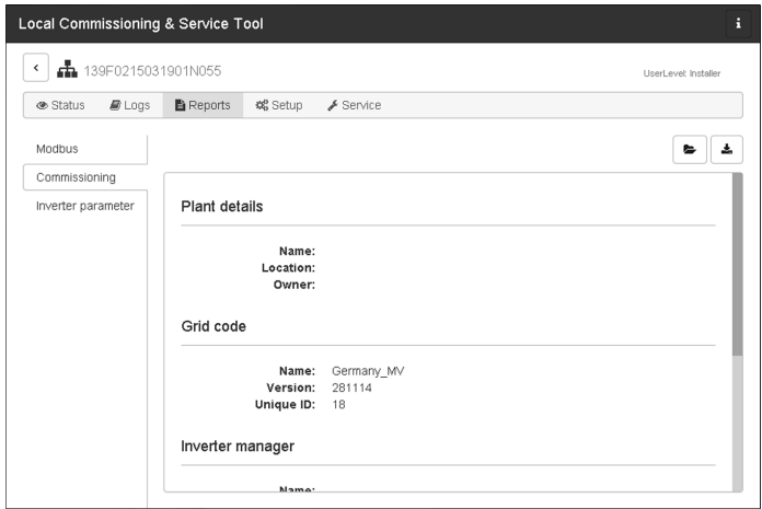
Abbildung 17: LCS-Tool - Inbetriebnahmebericht
