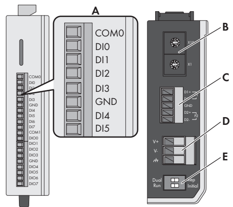
Imagen 9: Vista general de la conexión I/O Box
