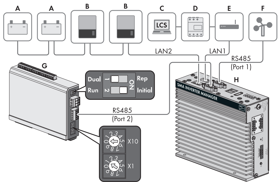
Figure 3:Vue d'ensemble du câblage Sunny Tripower Storage 60
