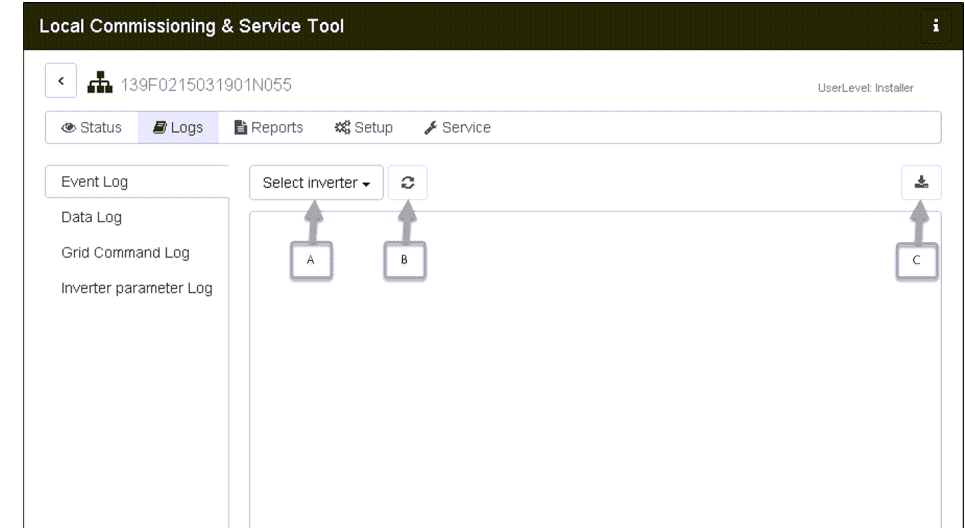
Abbildung 35: LCS-Tool - Logs
