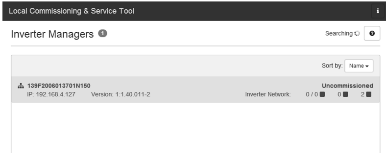
Abbildung 11: LCS-Tool - Startbildschirm
