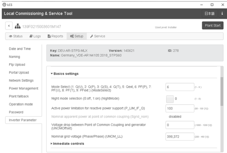
Figure 30:LCS-Tool - Activation/désactivation des paramètres onduleur
