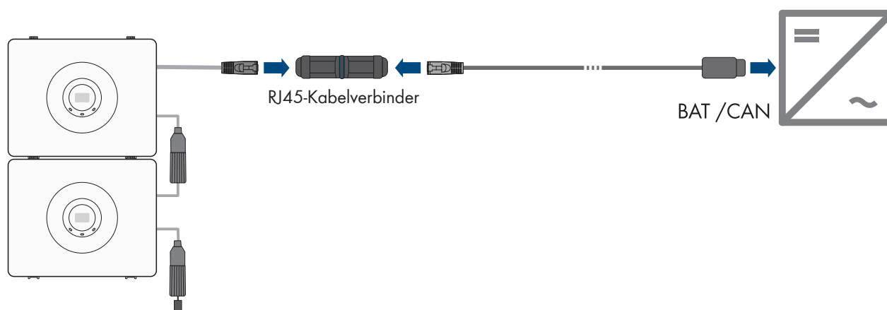
Abbildung 19: Anschlussübersicht der Batteriekommunikation mit dem Wechselrichter
