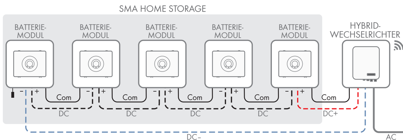
Abbildung 7: Modularer Aufbau der Batteriemodule
