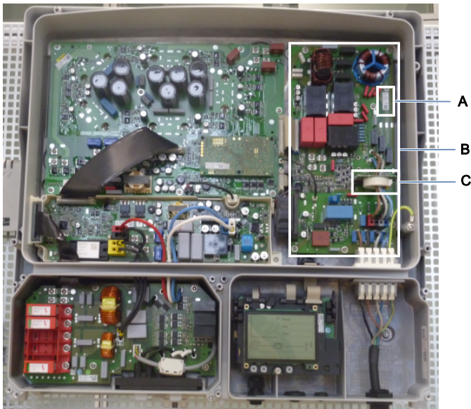
Abbildung 1 : Position im Wechselrichter
