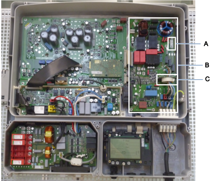
Afbeelding 1 : Positie in de omvormer
