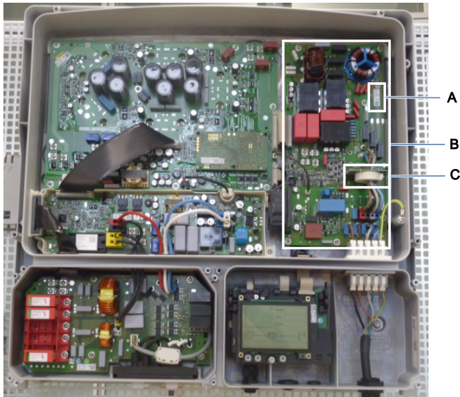
Figure 1 : Position dans l'onduleur
