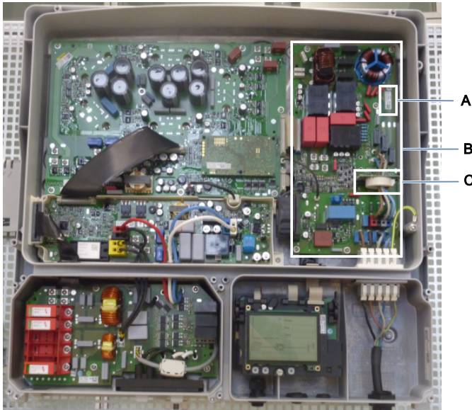
Imagen 1 : Posición en el inversor
