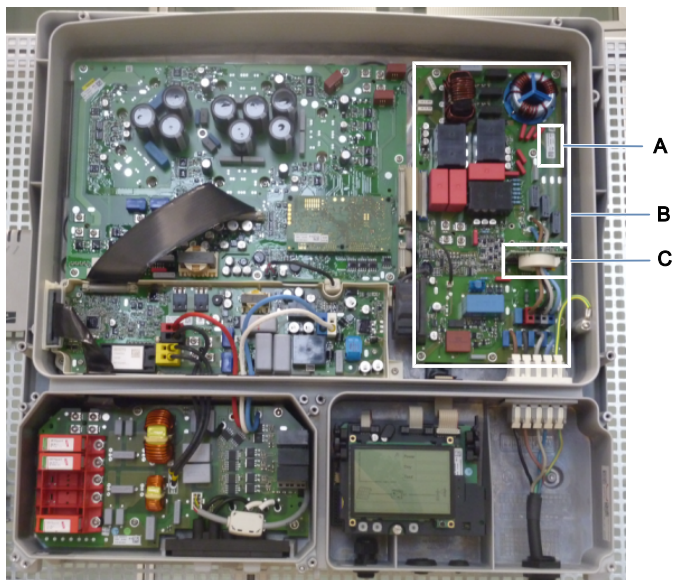
Figura 1 : Poziția în inverter
